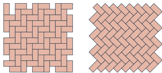
Elleboogverband
