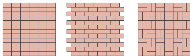
Steensverband
